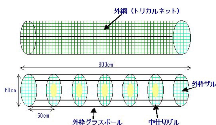
養殖カゴの模式図
