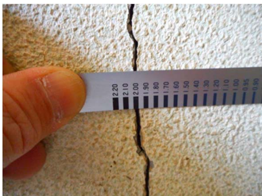
写真 亀裂幅の測定
