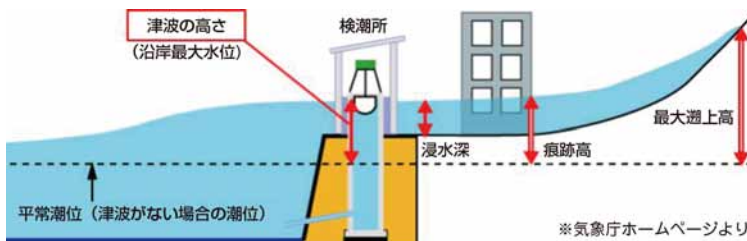
津波の高さと浸水深、痕跡高、遡上高の関係
